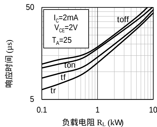
Fig.8 响应时间 vs 负载电阻曲线图
