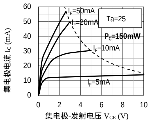
Fig.4 集电极电流 vs 集-发电压曲线图
