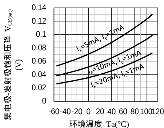
Fig.6 饱和压降 vs 环境温度曲线图
