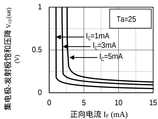
Fig.10 饱和压降 vs 正向电流曲线图
