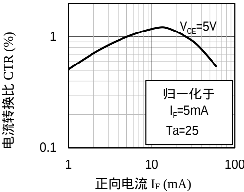
Fig.2 电流转换比 vs 正向电流曲线图
