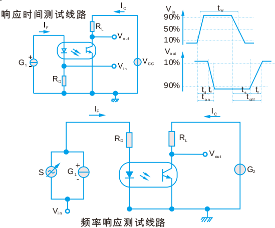
Fig.1 测试线路图
